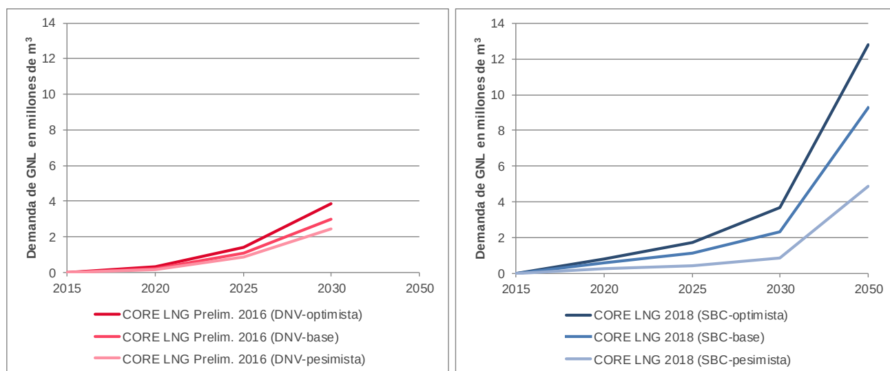
Figura III-5. Resumen de resultados de los estudios realizados para determinar el potencial de la demanda nacional de GNL en el transporte marítimo
